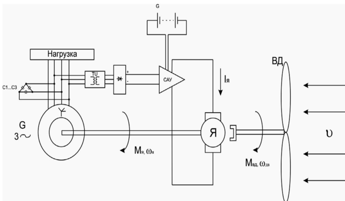
Рисунок 2.1– Электромеханическая схема ветроэнергетической установки:
