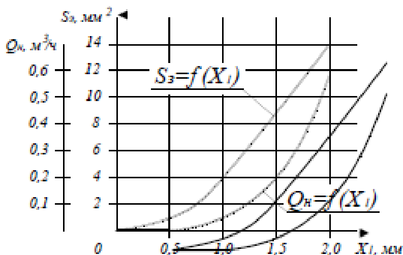
Рисунок 2.8 – Зависимости производительности Q_n и площади S_z от хода якоря X_l
